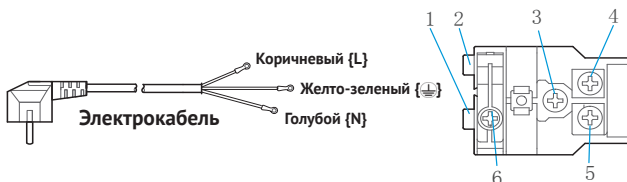
КЛЕММНАЯ КОРОБКА
